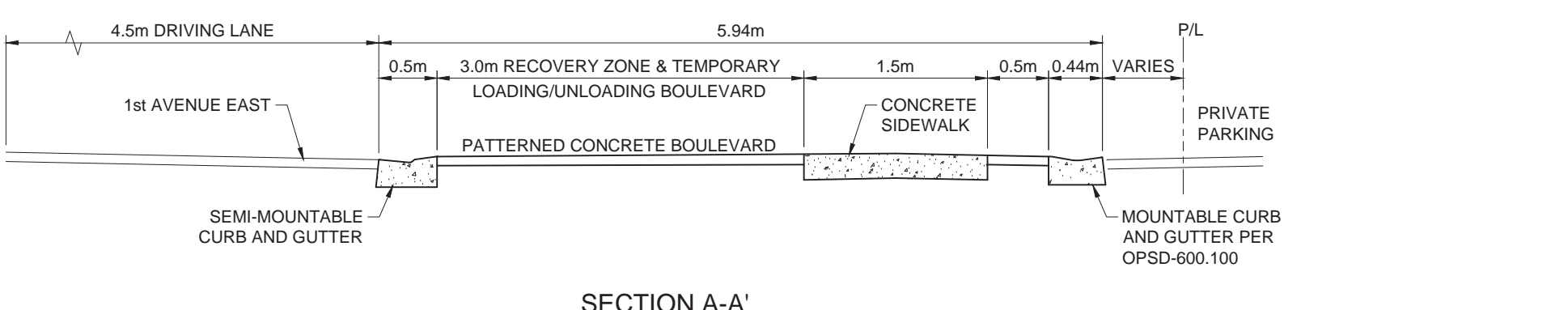
SECTION A-A'
